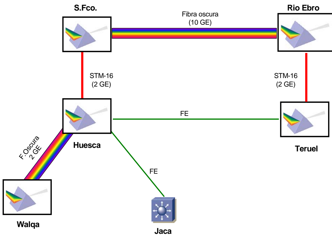
Figura 4.- Esquema de conexiones de la RIA (Red de Investigación de Aragón).
