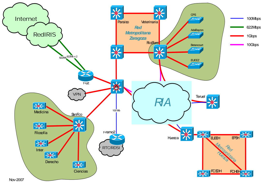
Figura 3.- Estructura de la Red Informática de la Universidad de Zaragoza.
