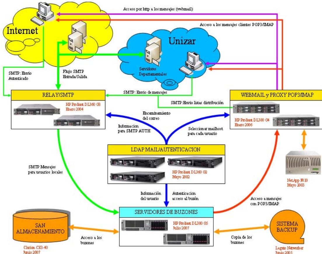
Figura 13.- Estructura informática del sistema de correo electrónico de la UZ.
