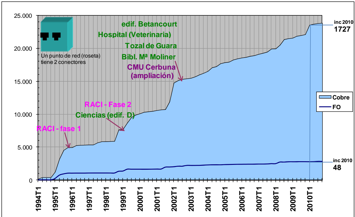
Figura 7.- Evolución del cableado estructurado de la Universidad de Zaragoza: conexiones en cobre y fibra óptica.
