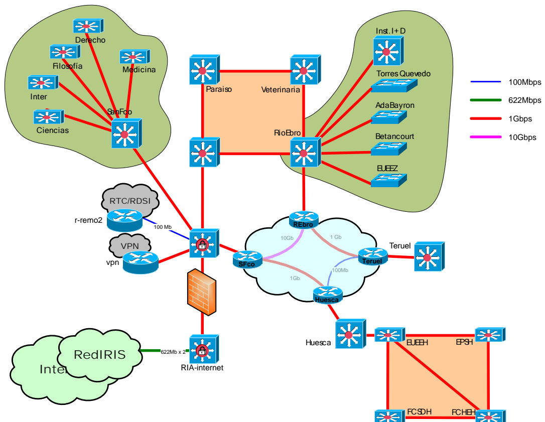
Figura 3.- Estructura de la Red Informática de la Universidad de Zaragoza.
