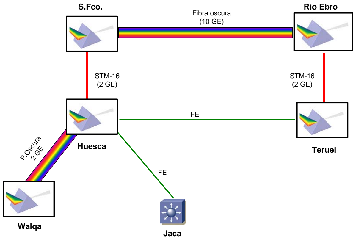
Figura 4.- Esquema de conexiones de la RIA (Red de Investigación de Aragón).
