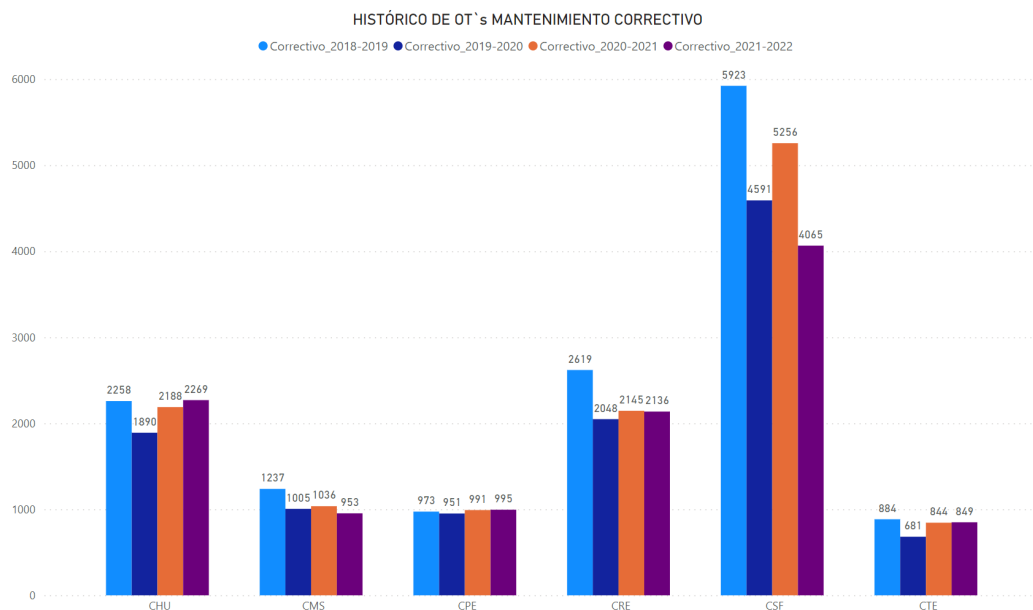
Figura: Evolución del número de OTs de Correctivo por Campus.
