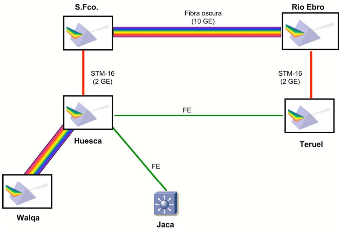
Figura 3. Esquema de conexiones de la RIA (Red de Investigación de Aragón).
