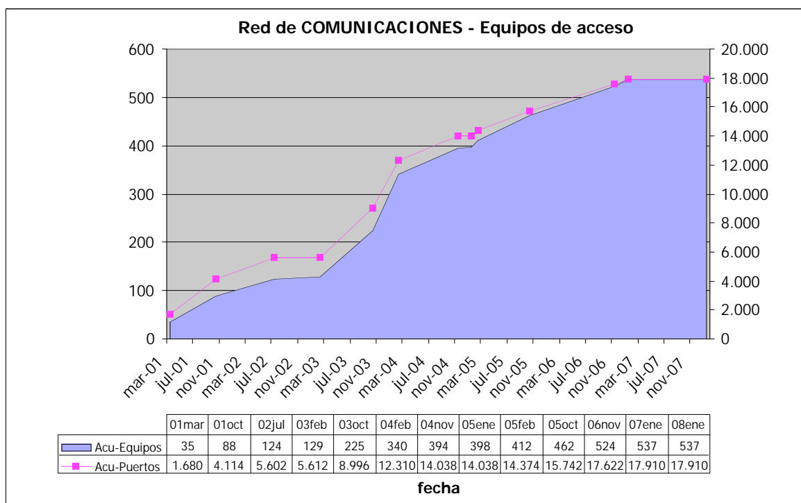
Figura 7. Equipos de comunicaciones desplegados en la Universidad, su evolución desde 2001 y el número de conexiones informáticas que proporcionan.
