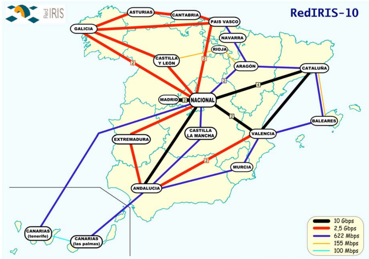
Figura 4. Estructura y conexiones de RedIRIS.
